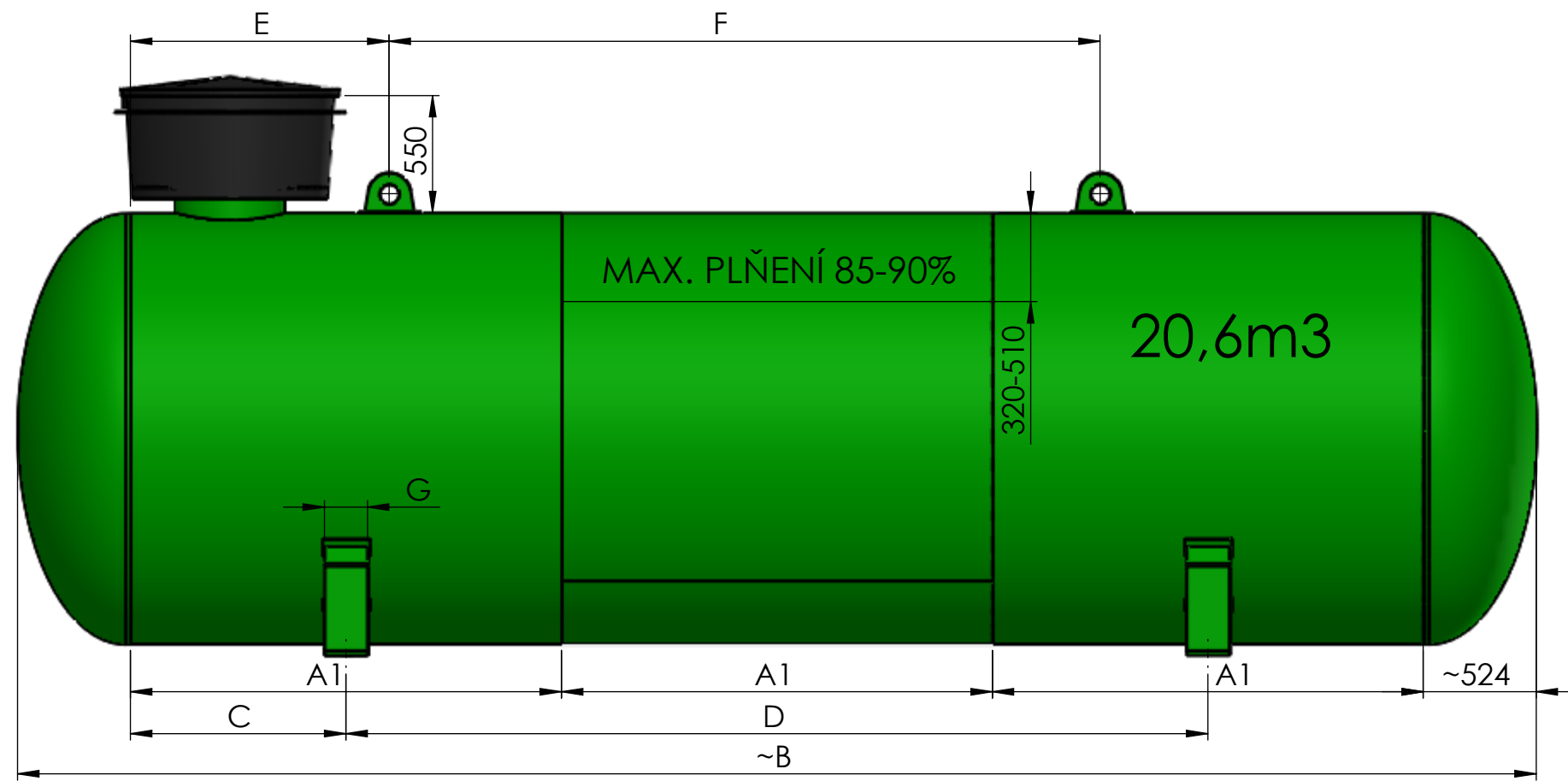
TABULKA OBJEMŮ A ZÁKLADNÍCH ROZMĚRŮ NÁDRŽÍ
